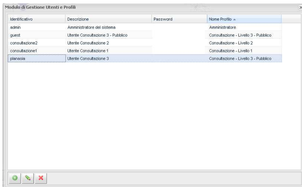
Figura 4 – Interfaccia per la gestione degli utenti
